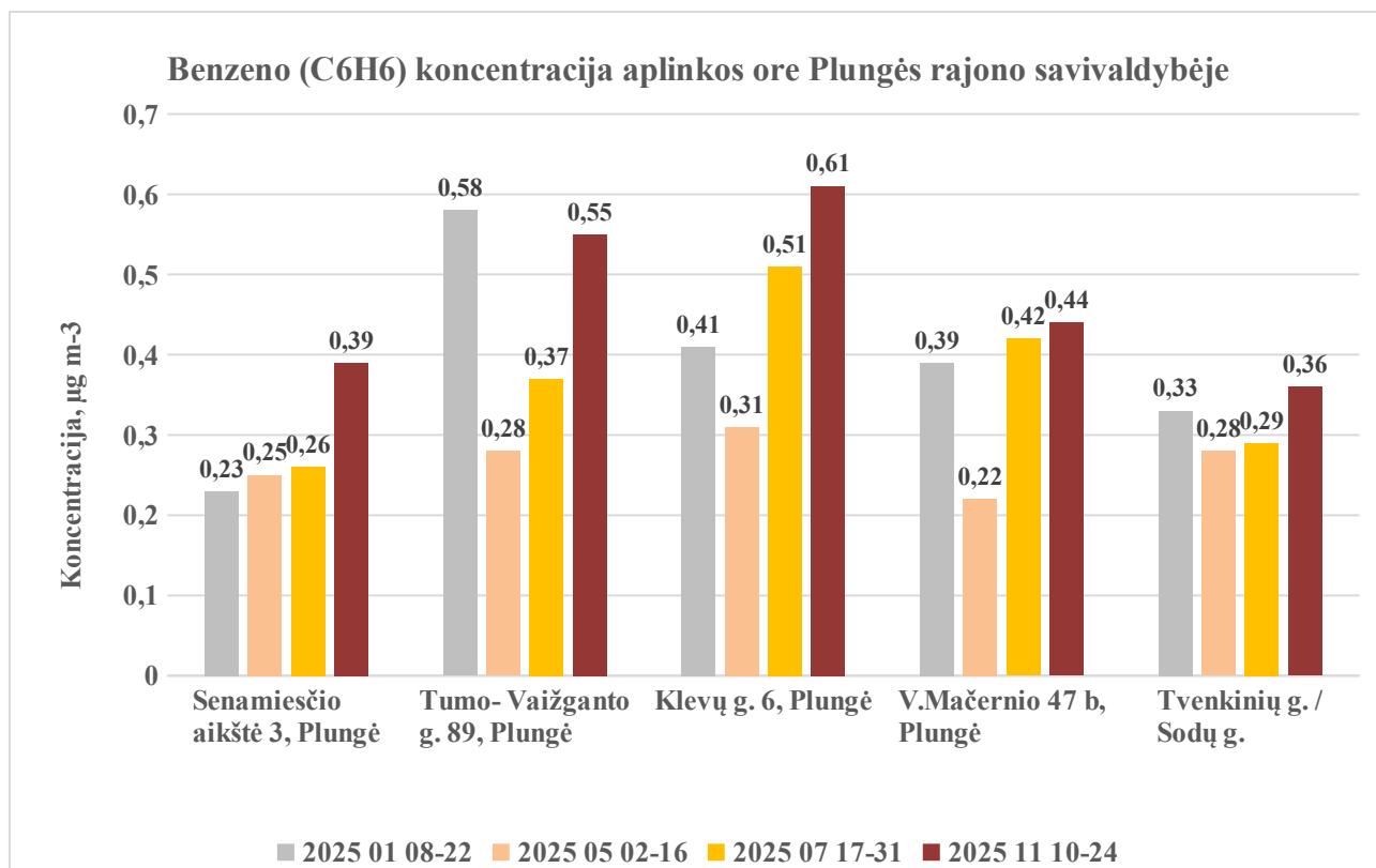
2.4 pav. Benzeno (C 6 H 6 ) koncentracija aplinkos ore Plungės rajono savivaldybės monitoringo taškuose 2025 m
