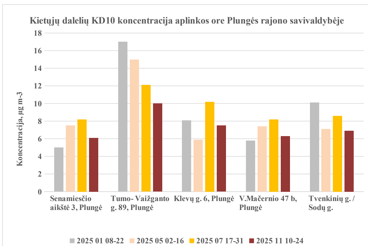
2.5 pav. Kietųjų dalelių ( KD_{10} ) koncentracija aplinkos ore Plungės rajono savivaldybės monitoringo taškuose 2025 m.
