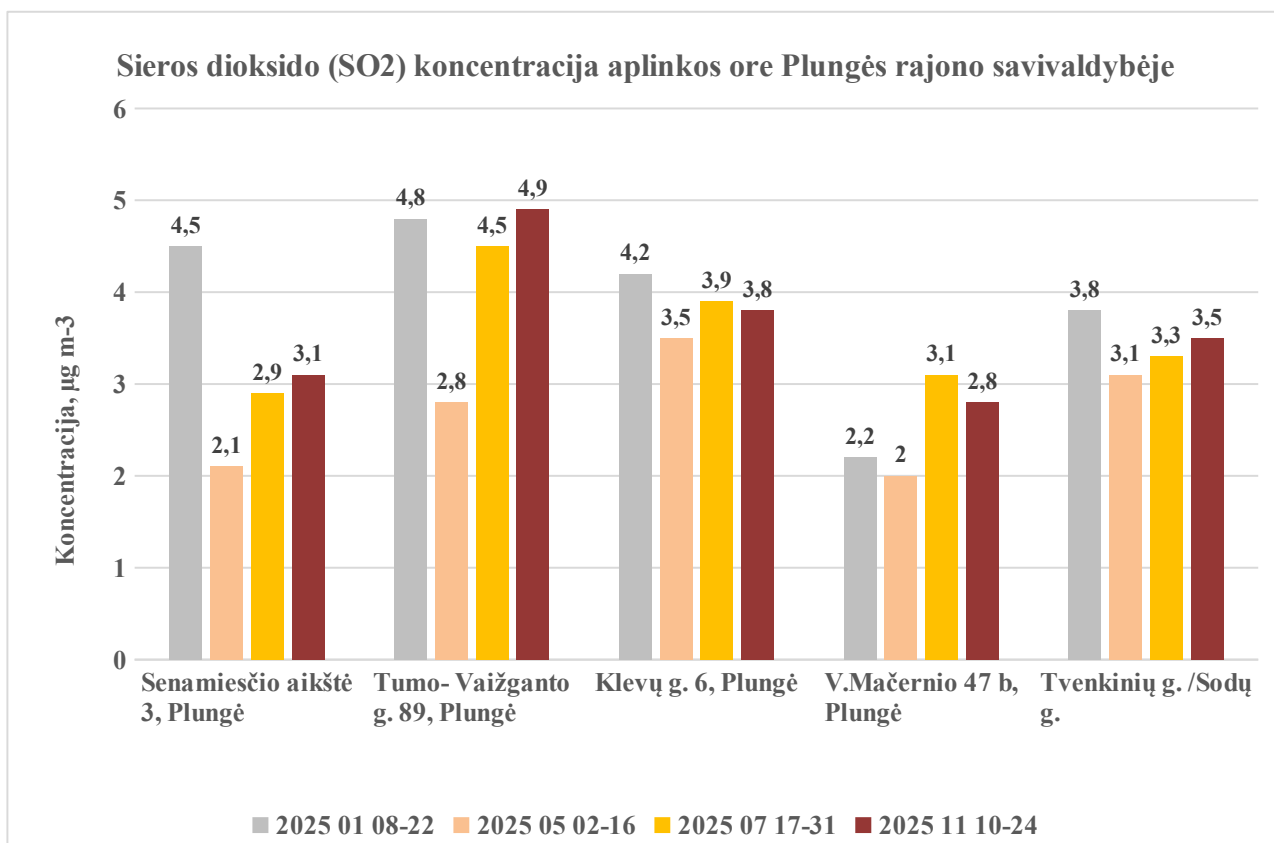
2.3 pav. Sieros dioksido (SO 2 ) koncentracija aplinkos ore Plungės rajono savivaldybės monitoringo taškuose 2025 m.
