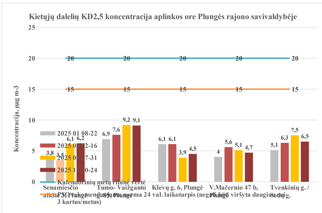
2.6 pav. Kietųjų dalelių ( KD_{2,5} ) koncentracija aplinkos ore Plungės rajono savivaldybės monitoringo taškuose 2025 m.
