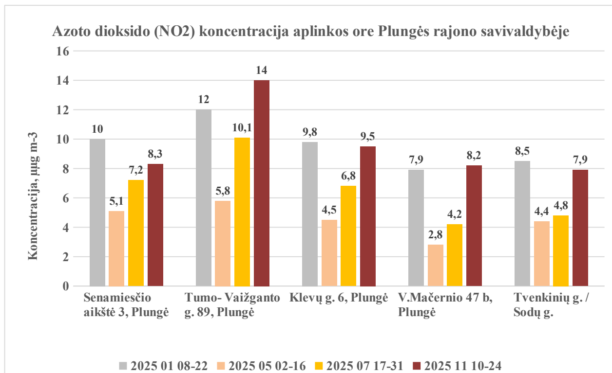
2.2 pav. Azoto dioksido (NO 2 ) koncentracijos Plungės rajono monitoringo vietose 2025 metais
