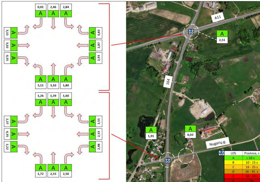
7 paveikslas. Eismo kokybės lygis ir gaisties laikas tinkle 2025 m. („Variantas 1“)
