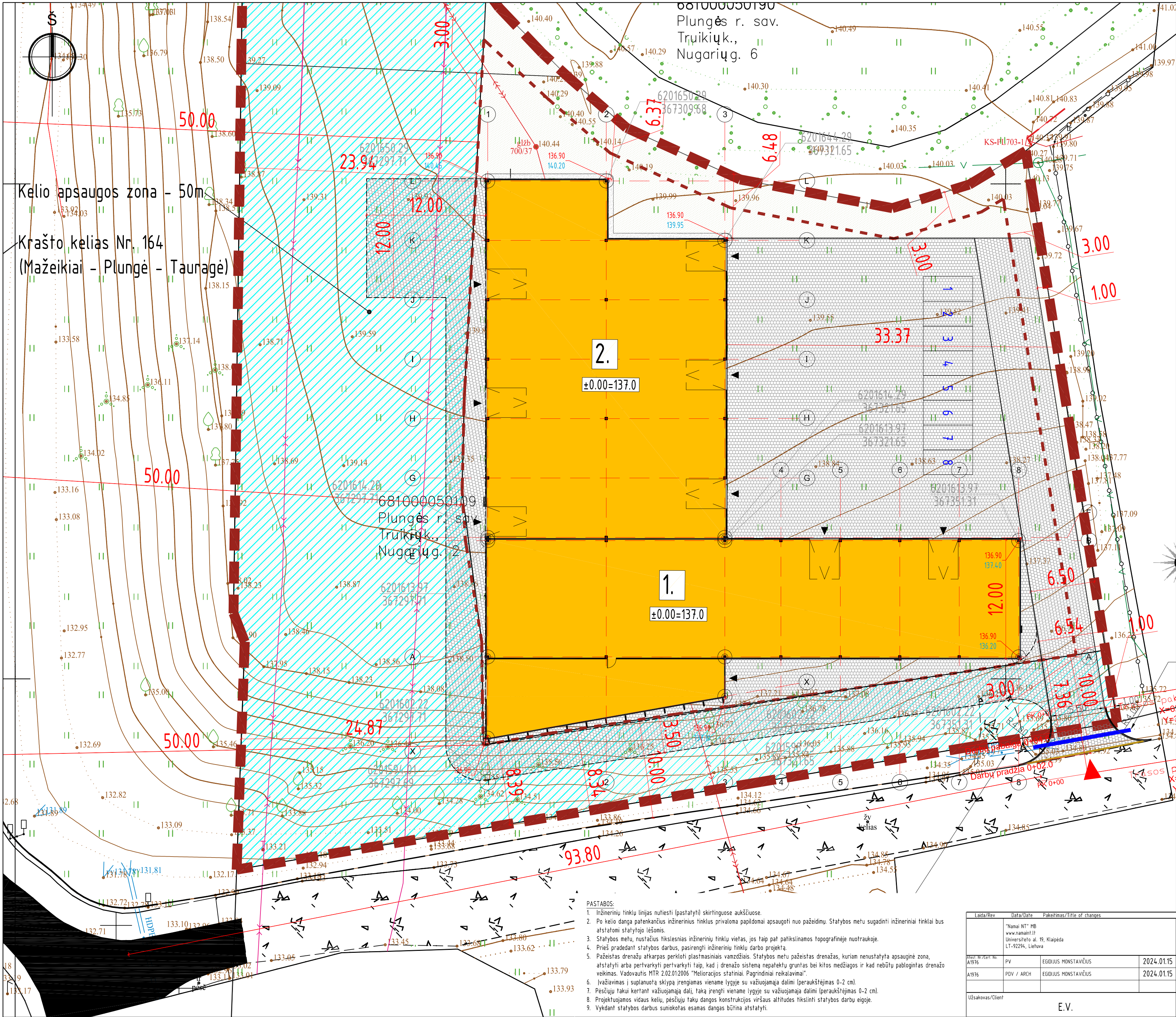
Viso sklypo plano Nugarių g. 2 schema
