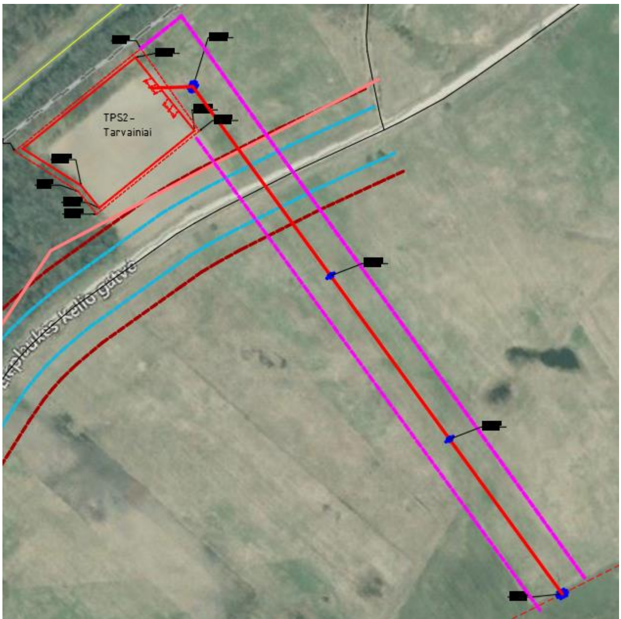
1 paveikslas. TPS2 prijungimas prie LITGRID tinklo
