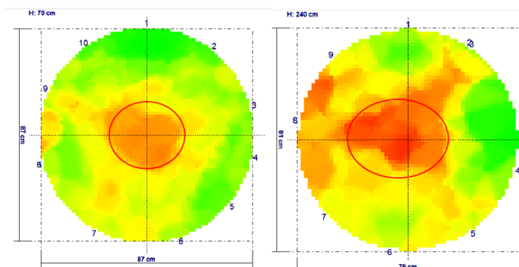
Akustinės tomografijos nuotraukos 0,7 ir 2,4 m aukštyje. Centrinio kamieno puvinio pažeista zona pažymėta raudonais apskritimais.
